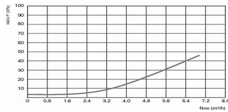
Druckverlust Rückflussverhinderer DN20:
