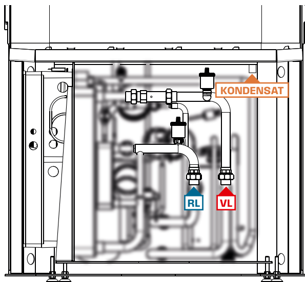
Abb. 16: Hydraulik anschließen
