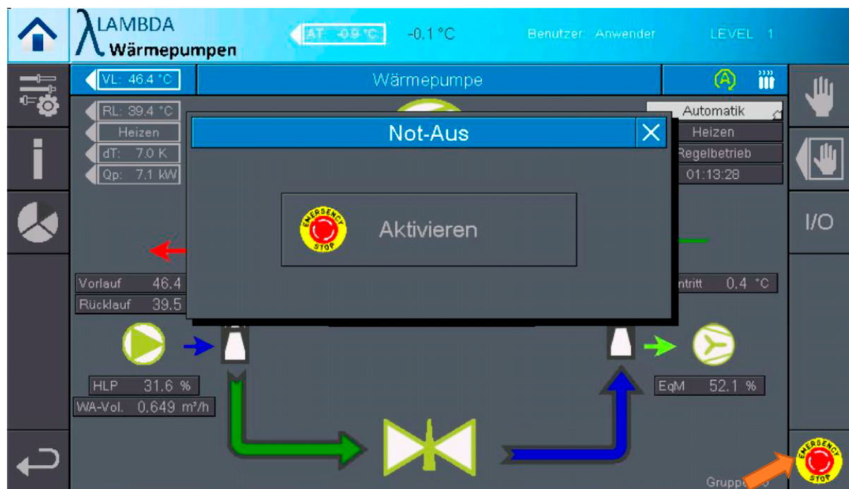
Abb. 23: Betriebsschalter
