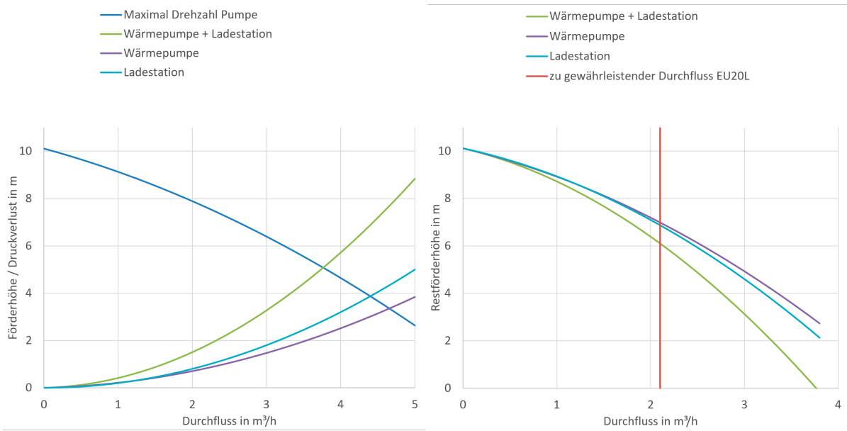
Abb. 17: Pumpenkennlinie, Anlagenkennlinie und Restförderhöhe EU20L
