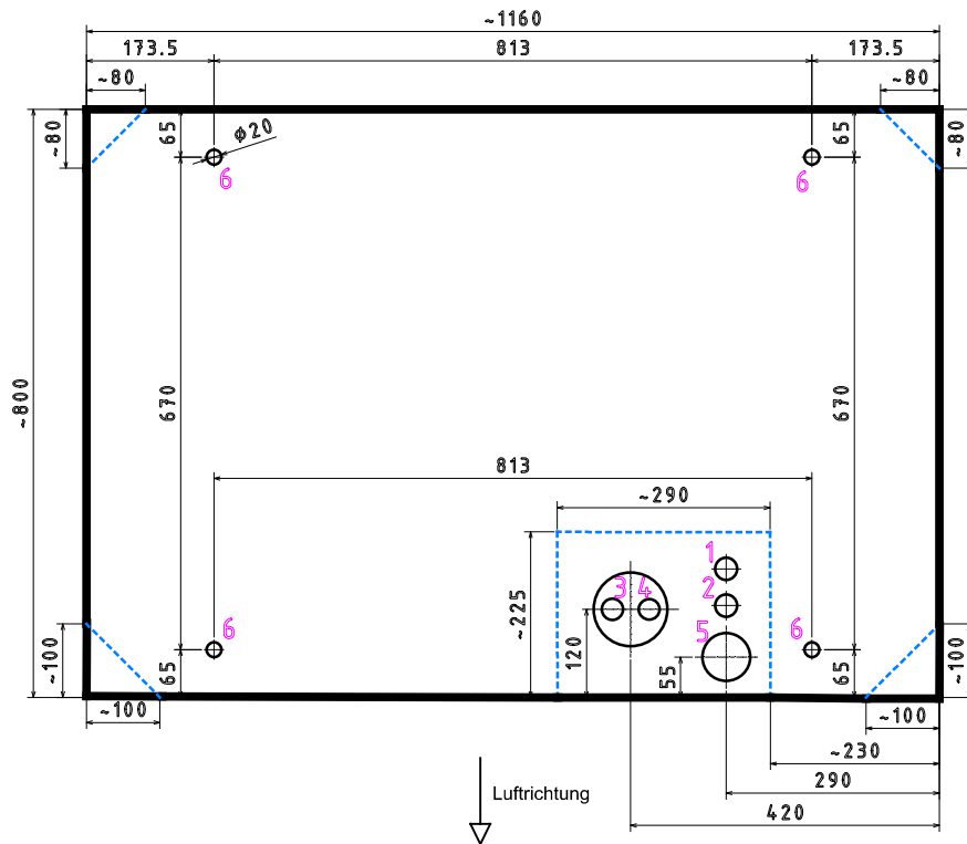
Draufsicht Sockel
