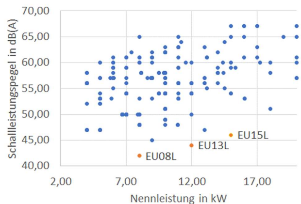
Marktvergleich Schalleistungspegel nach EN 12102
