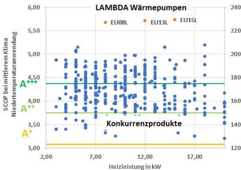
Marktvergleich Effizienz (SCOP) nach EN 14825
