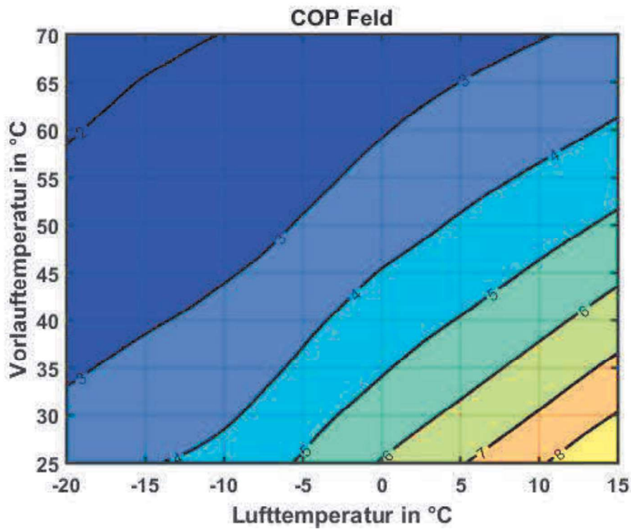
Abbildung 34: EU13L bei 9kW Heizleistung
