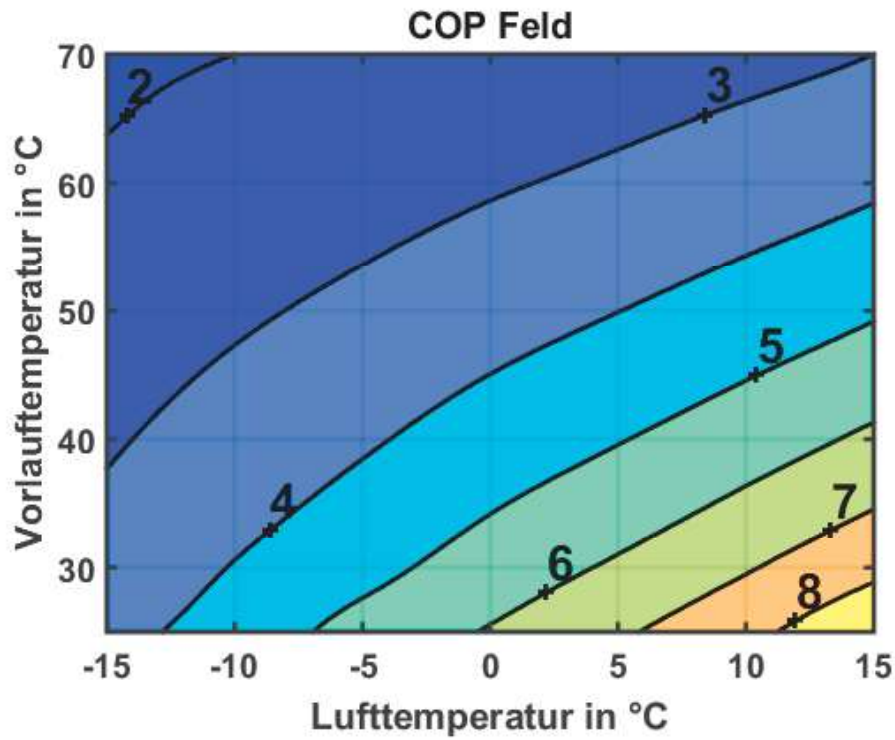
Abbildung 33: EU15L bei 12kW Heizleistung
