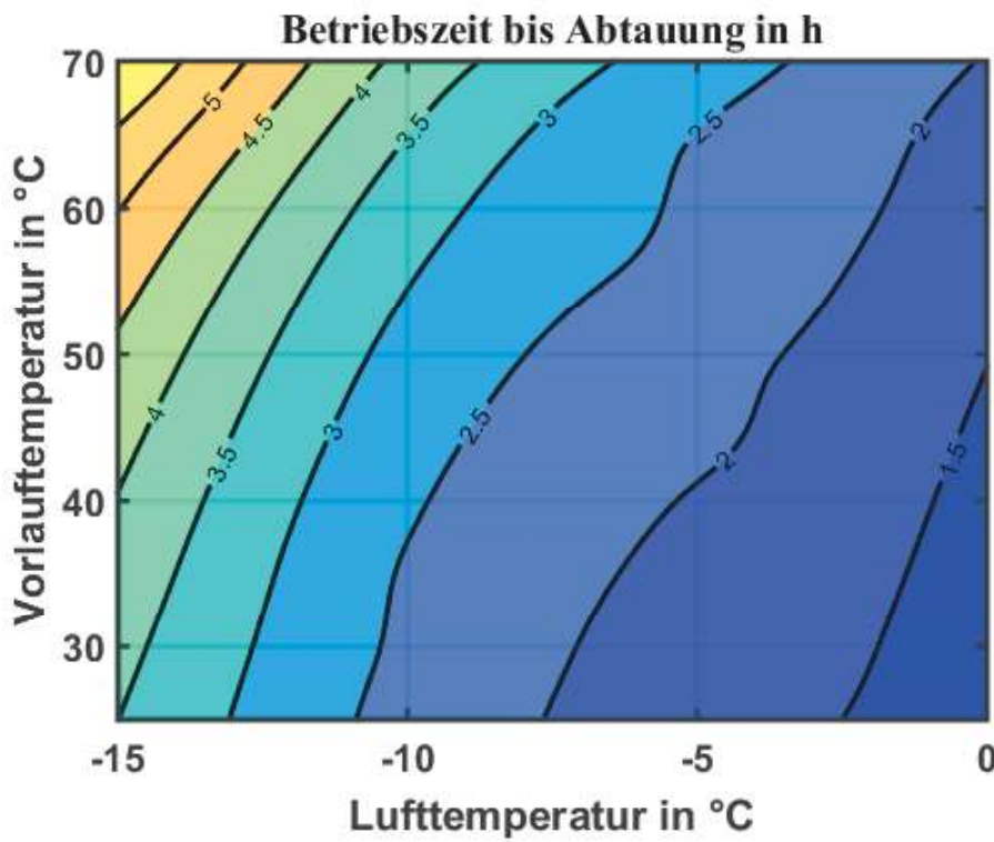
Abbildung 37: Betriebsdauer zwischen Abtauzyklen bei 9kW Heizleistung und 95% Luftfeuchte (EU13L)
