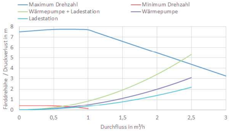
Abbildung 39: Pumpenkennlinie Grundfoss UPM3L 75/180 und Anlagenkennlinie
