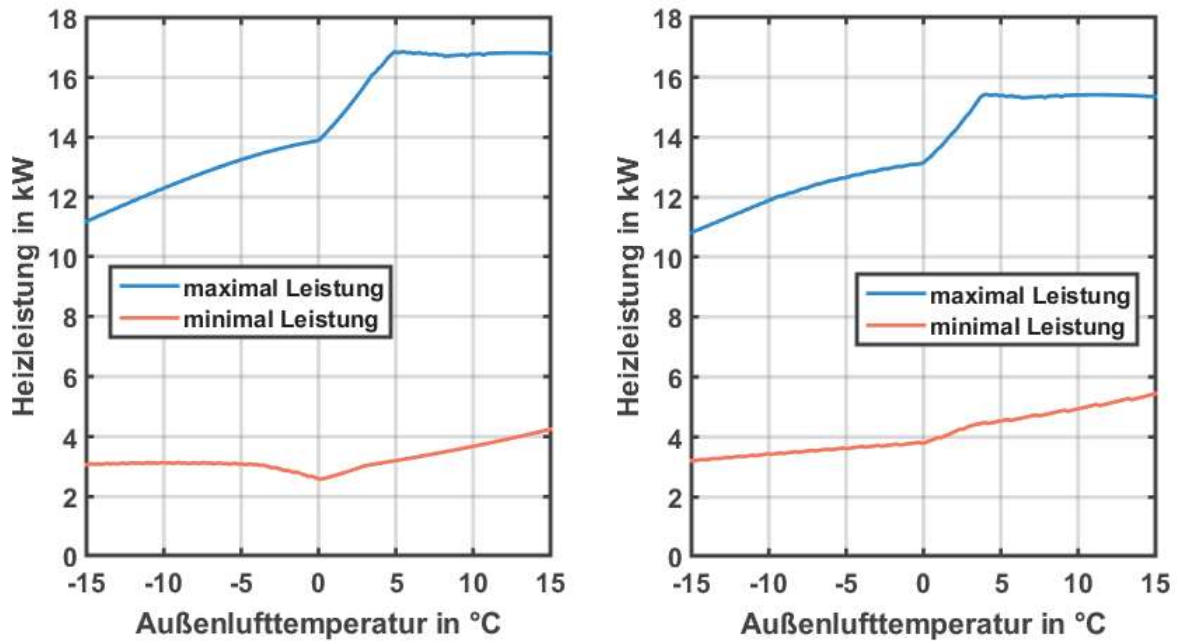
Abbildung 29: EU13L bei 5K Spreizung (links: 35°C Vorlauftemperatur / rechts: 55°C Vorlauftemperatur)
