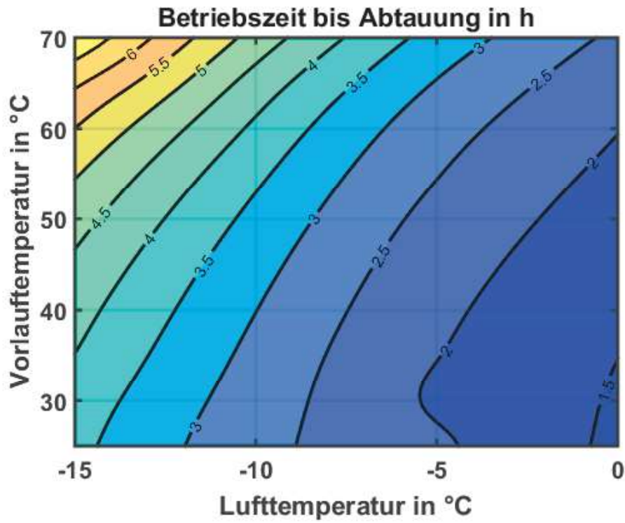
Abbildung 36: Betriebsdauer zwischen Abtauzyklen bei 9kW Heizleistung und 95% Luftfeuchte (EU15L)
