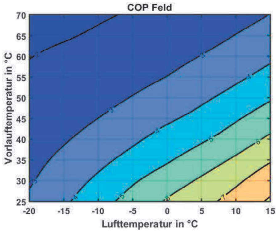
Abbildung 35: EU08L bei 6kW Heizleistung
