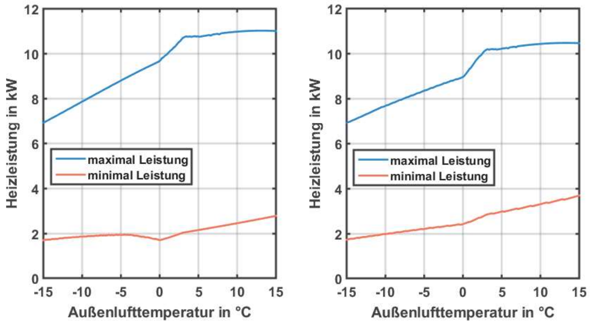
Abbildung 31: EU08L bei 5K Spreizung (links: 35°C Vorlauftemperatur / rechts: 55°C Vorlauftemperatur)
