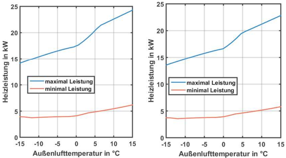
Abbildung 27: EU15L bei 5K Spreizung (links: 35°C Vorlauftemperatur / rechts: 55°C Vorlauftemperatur)
