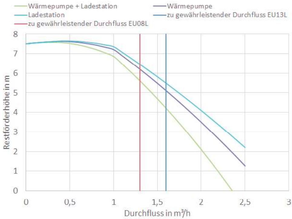
Abbildung 40: Restförderhöhe
