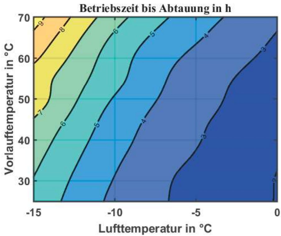
Abbildung 38: Betriebsdauer zwischen Abtauzyklen bei 6kW Heizleistung und 95% Luftfeuchte (EU08L)
