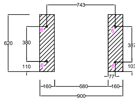
Draufsicht Sockel
